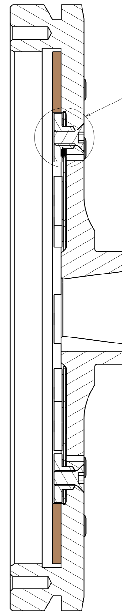
Section view A-A Scale: 1:1
